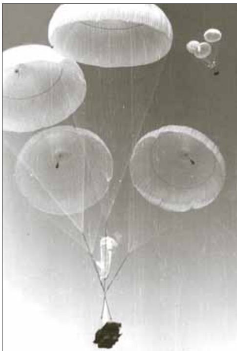
Padáková plošina P-127 s vozidlem GAZ a bezzákluzovým kanonem se snáší k zemi
